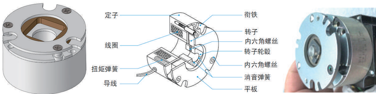
结构3D图
