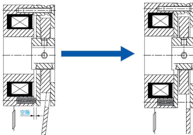
断电释放
