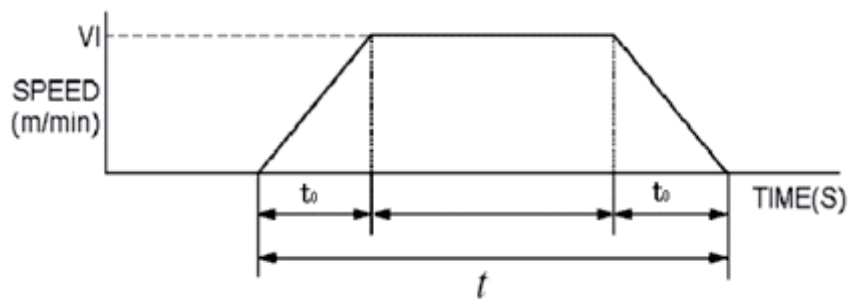
图3：运行曲线
