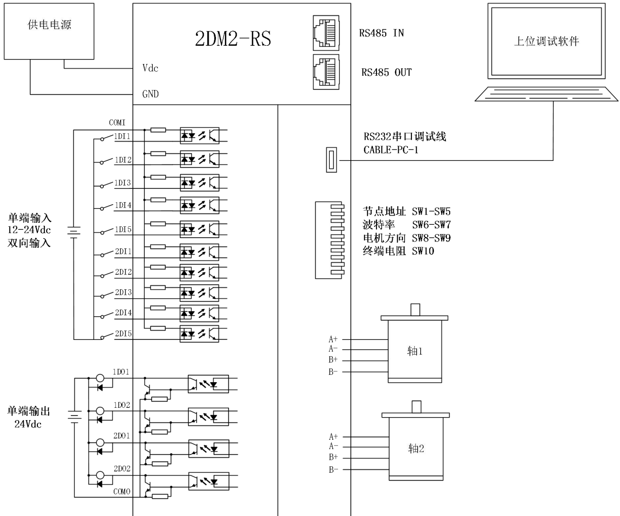
图 3-1 总线步进配线图
