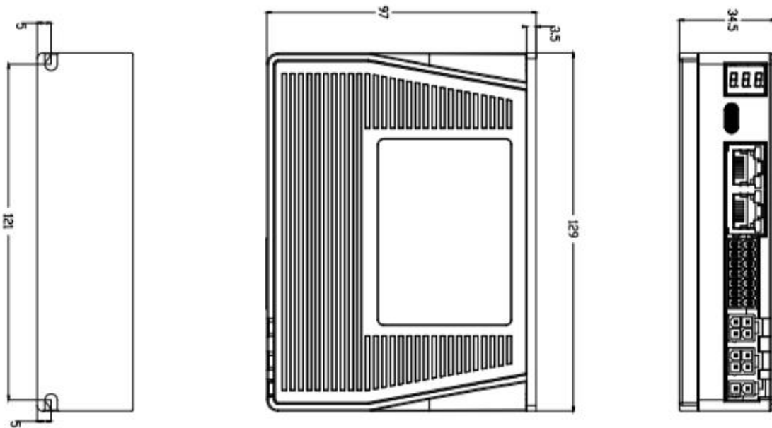
2DM3-EC556S: 长*高*宽: 129*97*34 (mm)
