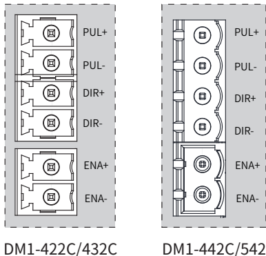
图 3-11 控制信号 /IO 端口示意图
