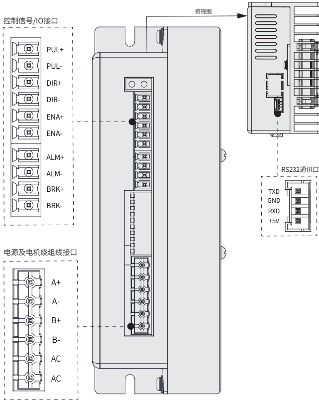
图 3-8 驱动器端子分布示意图
