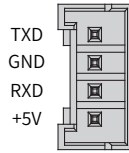
图 3-13 RS232 通讯端口示意图
