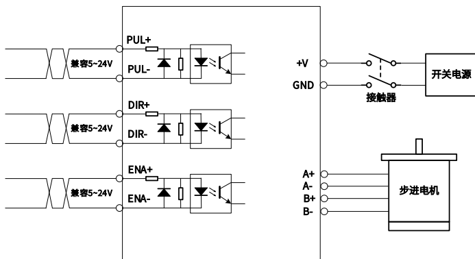
图 3-4 电气接线示意图
