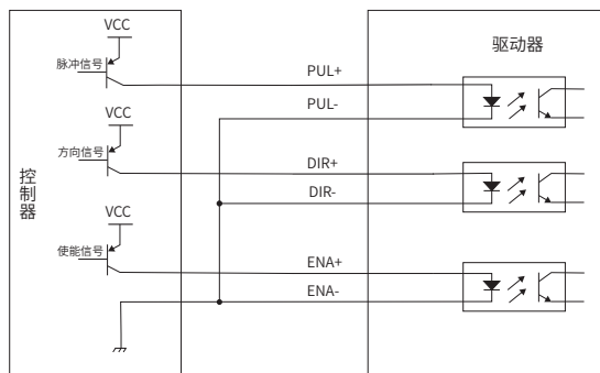
图 3-14 单端方式共阳极接法示意图
