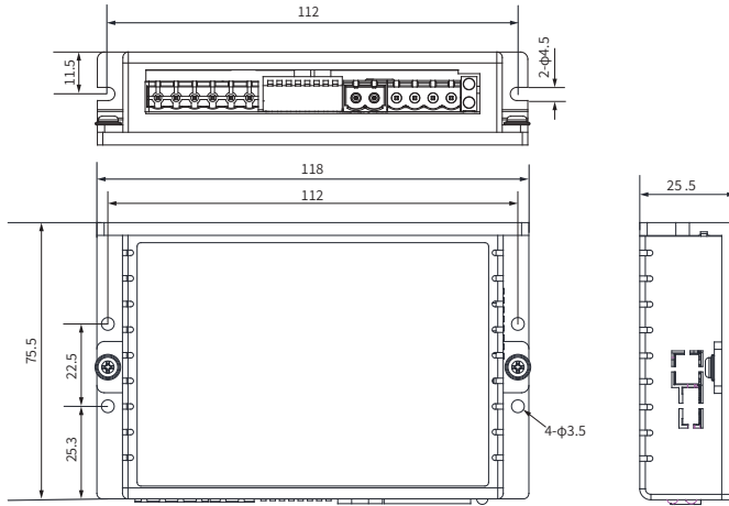
图 2-3 驱动器安装尺寸图 (单位: mm)
