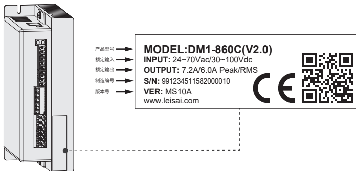
图 1-2 驱动器铭牌示例图 (DM1-860C 机型)
