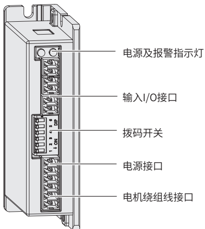
图 1-3 驱动器外观及部件示意图
