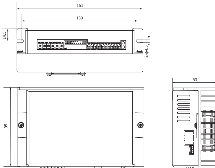
图 2-4 驱动器安装尺寸图 (单位: mm)
