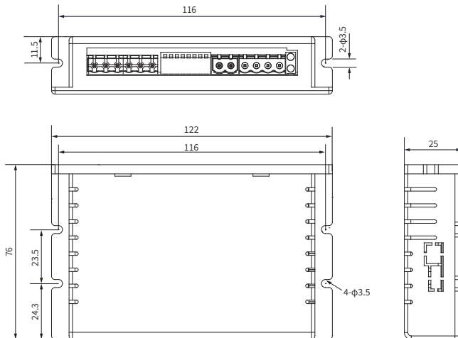
图 2-2 驱动器安装尺寸图 (单位: mm)
