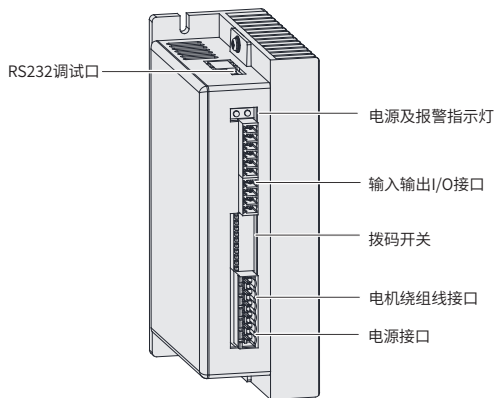
图 1-5 驱动器外观及部件示意图
