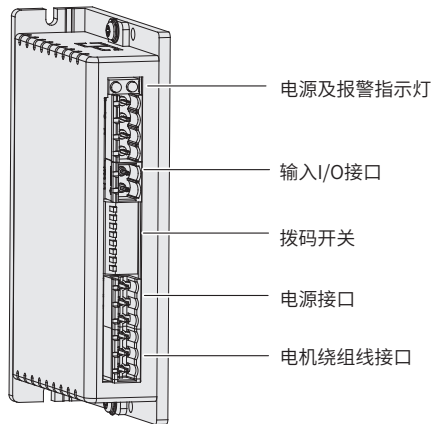
图 1-4 驱动器外观及部件示意图
