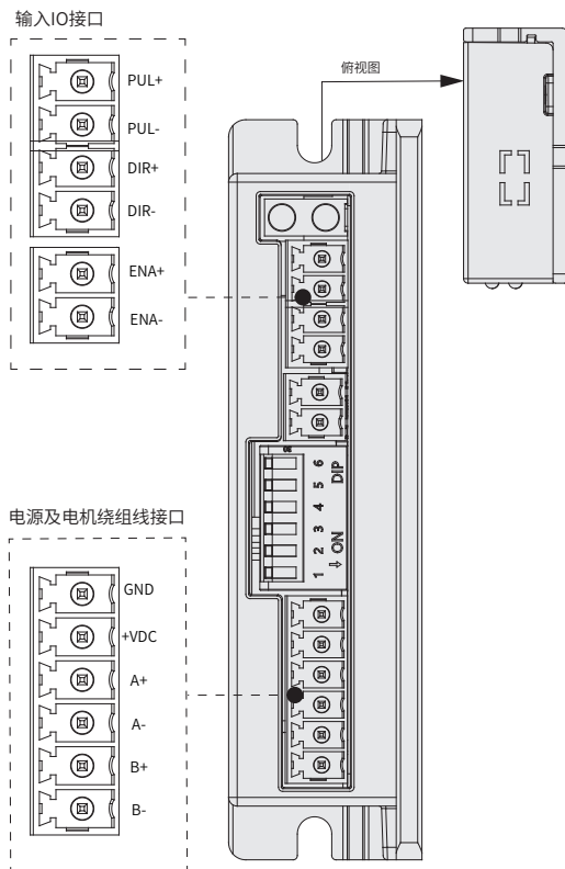
图 3-6 驱动器端子分布示意图
