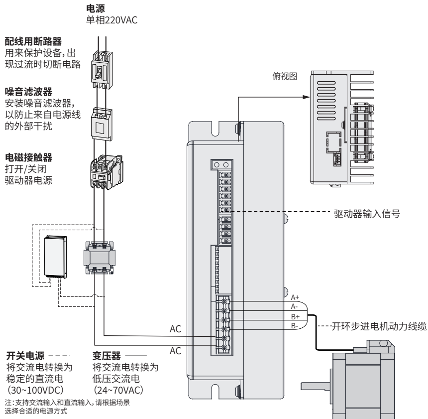
图 3-3 驱动器系统接线图
