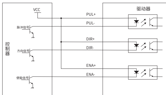
图 3-14 单端方式共阳极接法示意图
