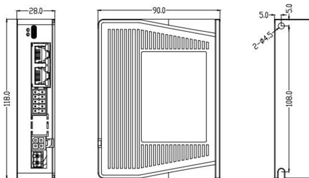
图 2-1 DM3B-EC522/542/556/570 安装尺寸图(单位: mm)
