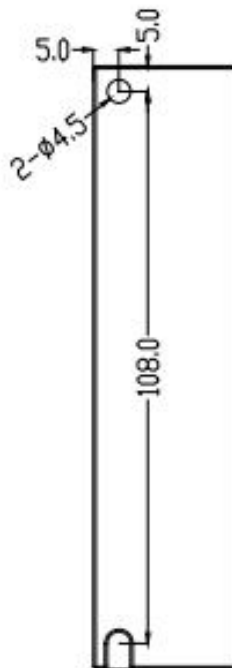
图 2-1 DM3B-EC522/542/556/570 安装尺寸图(单位: mm)
