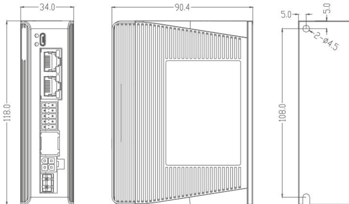
图 2-1 DM3C-522/556/870 安装尺寸图(单位: mm)
