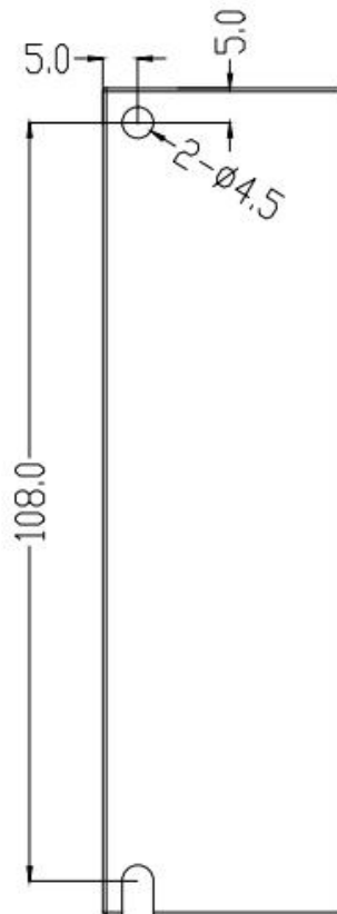
图 2-1 DM3C-522/556/870 安装尺寸图(单位: mm)
